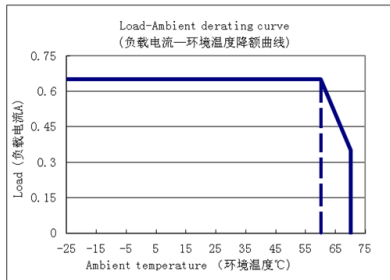
降额曲线图 (24V 输出电压):
