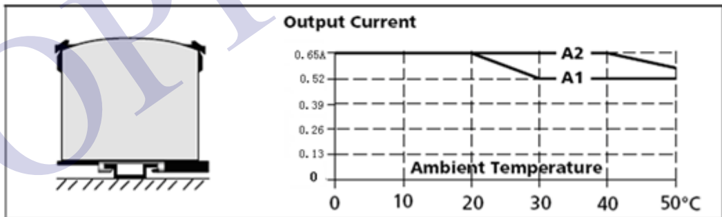
图 3-1 安装方向 C (桌面安装) (24V 输出电压)
