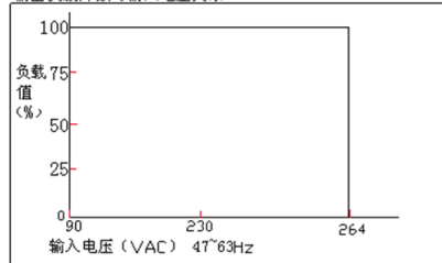
输出负载降额与输入电压关系
