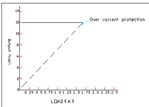
输出特性曲线 (12V输出电压):
