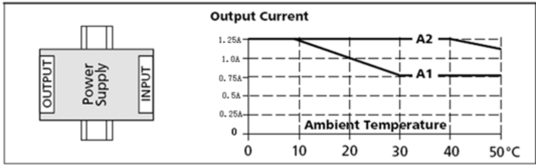
图 5-1 安装方向 E (水平安装方向) (12V 输出电压)
