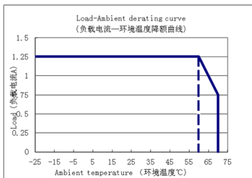
降额曲线图 (12V 输出电压):
