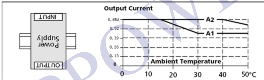
图 2-1 安装方向 B (倒转方向) (24V 输出电压)
