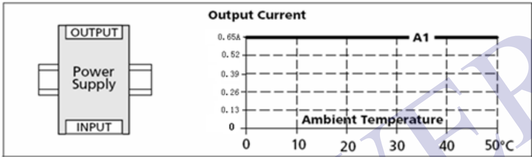
图 1-1 安装方向 A (标准安装方向) (24V 输出电压)
